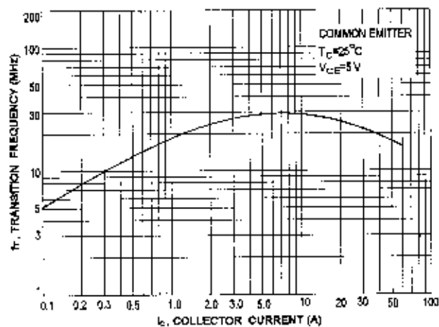
f_T - I_C
