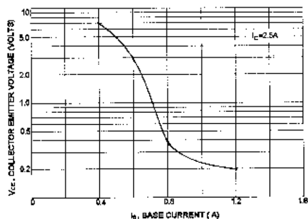
V_{CE(sat)} - I_B
