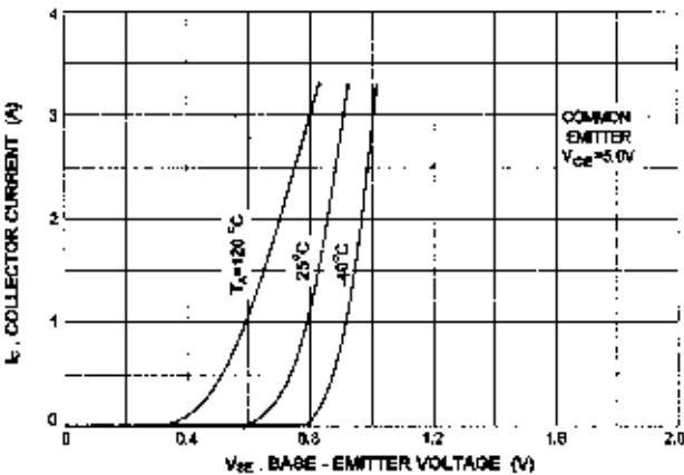
I_C - V_{BE}
