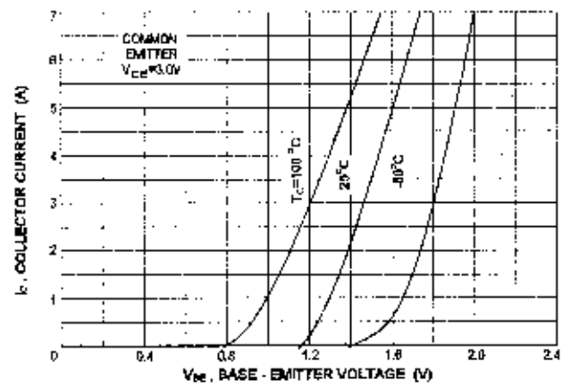
IC - VBE
