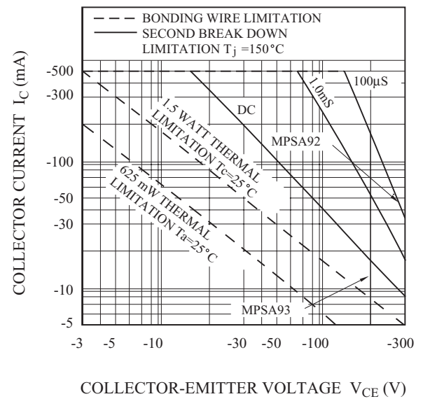
I_C - V_{CE}
