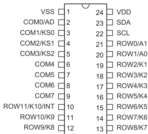
HT16K33 24 SOP-A
